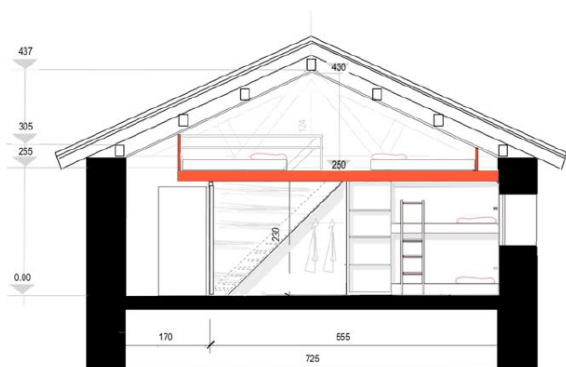
SEZIONE A-A
